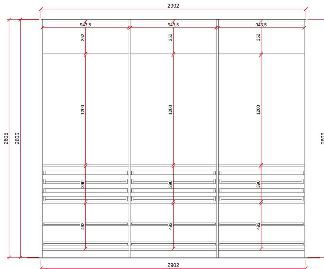
VISTA D - ESC. 1:25
