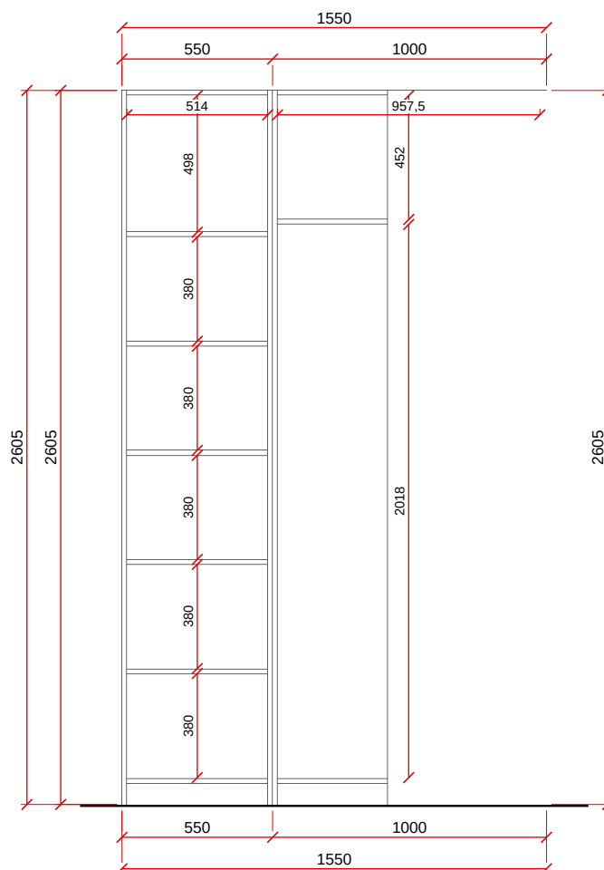
VISTA C - ESC. 1:25
